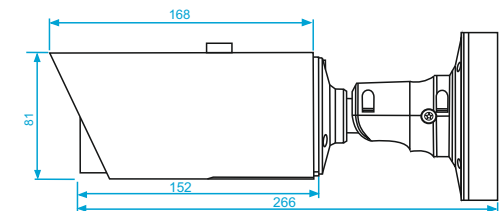
Rysunek techniczny
